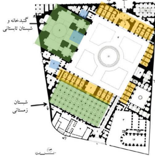
پلان مسجد - مدرسه سپهسالار جدید
