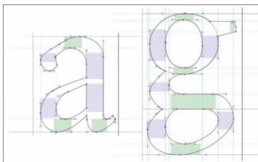
شکل ۲: استفاده از منحنی‌های بزیه در طراحی حروف.
