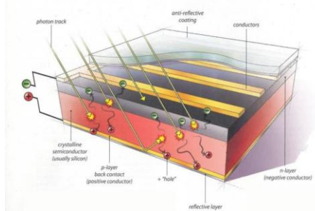
شکل ۱- طرح کلی از یک سلول خورشیدی (۷)
