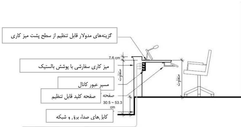
شکل ۲ طرح مقطع جایگاه نشست قاضی (منبع: نشریه ۷۸۱ ص ۹۰)
