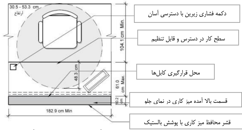
شکل ۱ طرح پلان جایگاه نشست قاضی (منبع: نشریه ۷۸۱ ص ۸۹)
