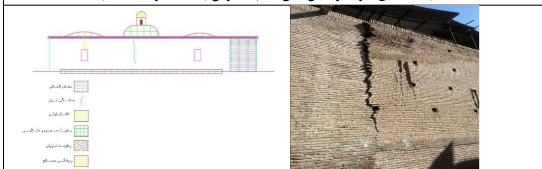
شکل ۱۲- نمای دیوار مسجد و نشان دادن آسیب ها در آن (مأخذ: نگارنده ۱۴۰۲)
