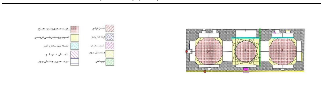
شکل ۱۴- تحلیل آسیب گنبد خانه مسجد مدرسه سردار (مأخذ: نگارنده ۱۴۰۲)
